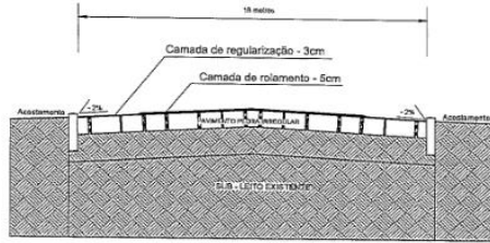
SEÇÃO TRANSVERSAL TIPO Esc. 5cm escala
