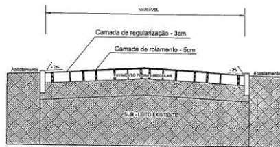
SEÇÃO TRANSVERSAL TIPO Esc: Sem escala
