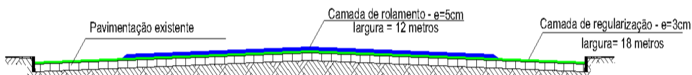
Imagem 05: Seção tipo
